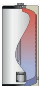
Edelstahldoppelmantelspeicher mit 2 Heizungsanschlüssen
